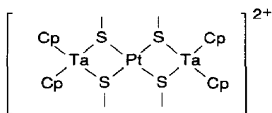
Fig. 29. Structure of 7.51 .
